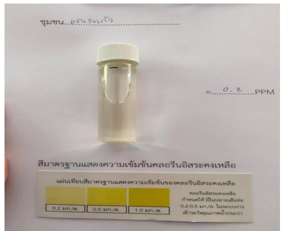
ชุมชนเณรแก้ว มีปริมาณคลอรีนอิสระคงเหลือในน้ำประปา ๐.๒ มิลลิกรัมต่อลิตร
