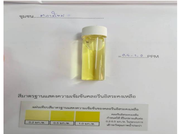
ชุมชนตลาดใหม่ มีปริมาณคลอรีนอิสระคงเหลือในน้ำประปา ๐.๕ - ๑.๐ มิลลิกรัมต่อลิตร
