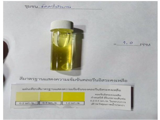
ชุมชนวัดศรีบัวบาน มีปริมาณคลอรีนอิสระคงเหลือในน้ำประปา ๑.๐ มิลลิกรัมต่อลิตร
