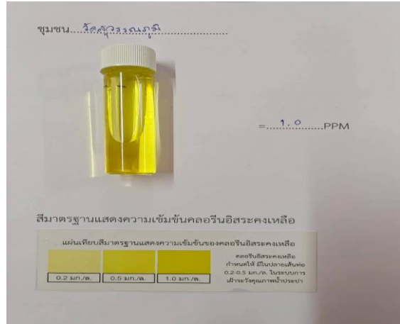
ชุมชนวัดสุวรณภูมิ มีปริมาณคลอรีนอิสระคงเหลือในน้ำประปา ๑.๐ มิลลิกรัมต่อลิตร
