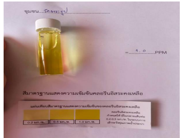
ชุมชนวัดพระรูป มีปริมาณคลอรีนอิสระคงเหลือในน้ำประปา ๑.๐ มิลลิกรัมต่อลิตร
