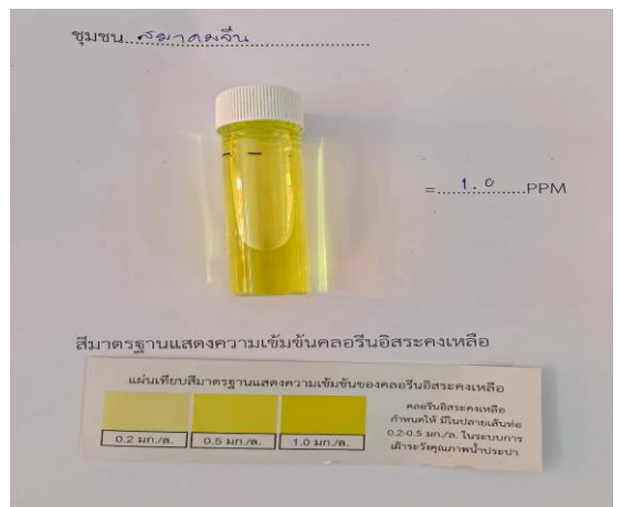
ชุมชนสยามคจีน มีปริมาณคลอรีนอิสระคงเหลือในน้ำประปา ๑.๐ มิลลิกรัมต่อลิตร
